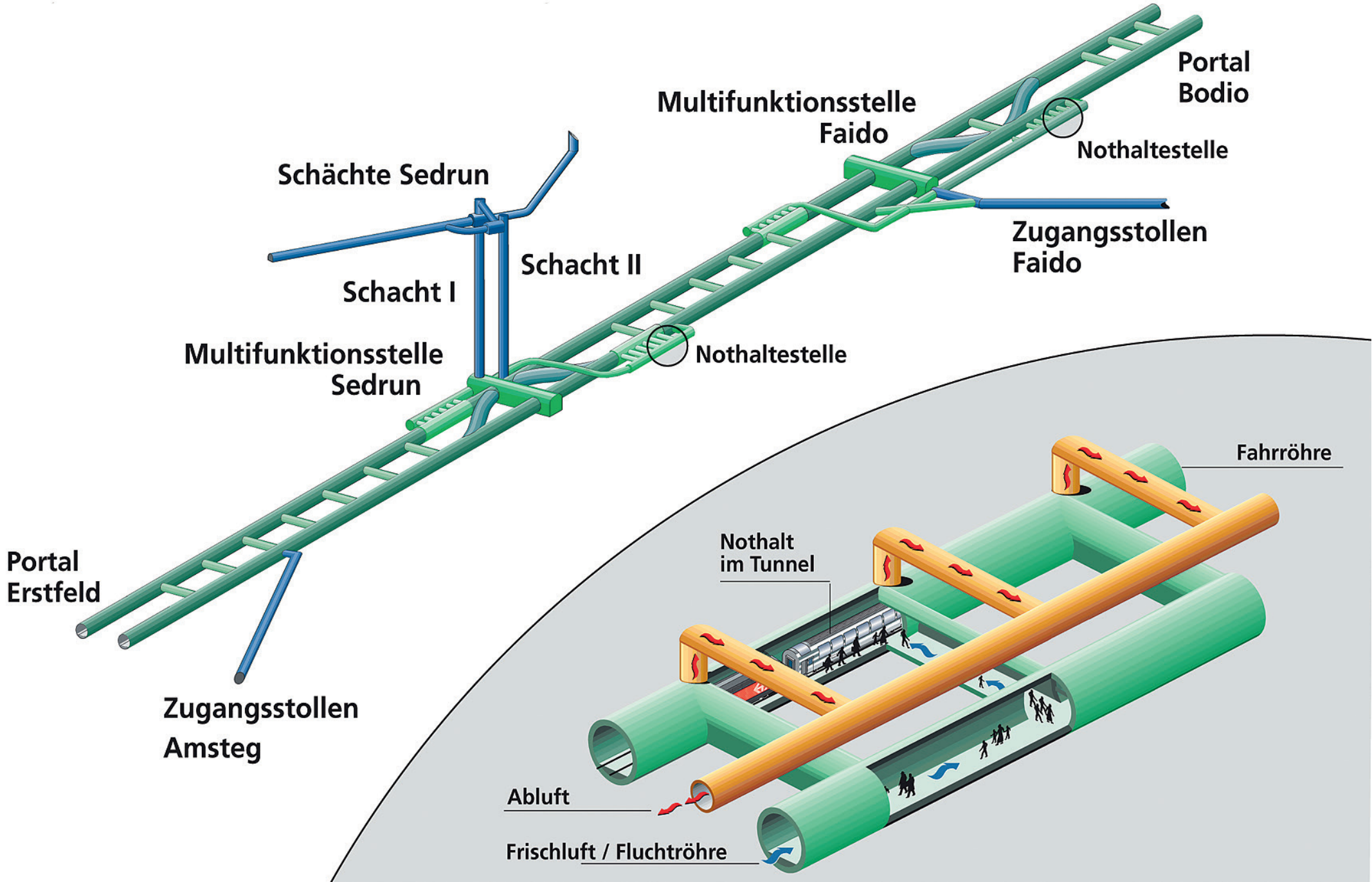
Schema Gotthard-Basistunnel. Quelle Alptransit
